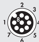
Vista dall'alto del connettore del regolatore
